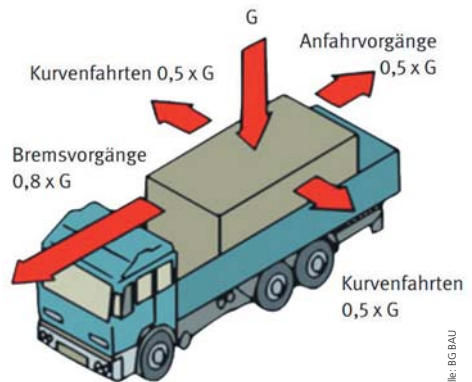
Massekräfte im Fahrbetrieb bei Fahrzeugen > 3,5 t
